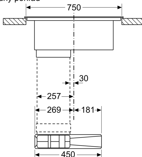
rozмеры в мм predný pohľad
