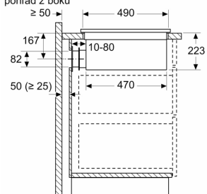
rozмеры в мм пohľad z boku
